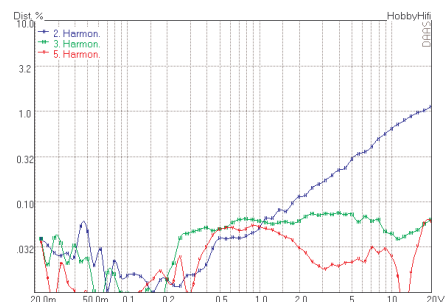
Klirrfaktor K2, K3 und K5 über Signalpegel bei 600 Hz Vom Kleinsignalbereich bis zu größter Lautstärke hervorragend.
