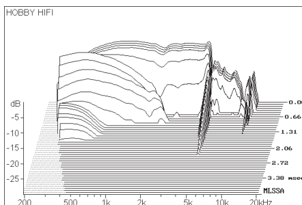
Wasserfallspektrum in unendlicher Schallwand axial Resonanzstelle bei 5 kHz mit langem Nachschwingen, darunter fehlerfrei.
