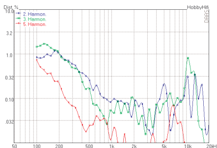
Klirrfaktor-Frequenzgänge K2, K3 u. K5 bei 90 dB mittlerem Schalldruckpegel Schon ab 500 Hz ausgesprochen niedrige Klirrwerte.
